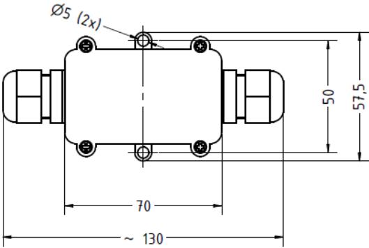
Pohled zepředu
